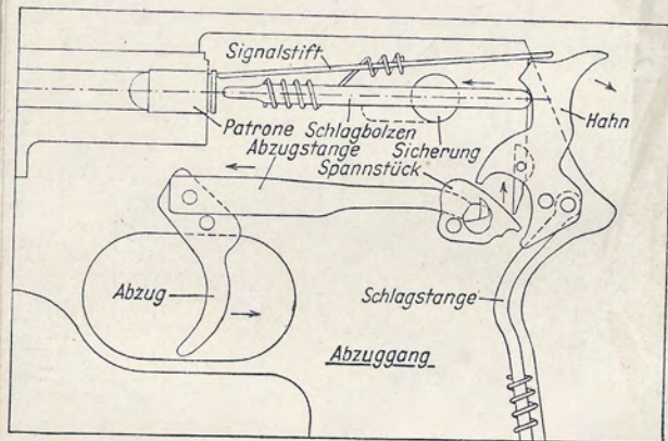
Abzugsgang der Pistole 38
