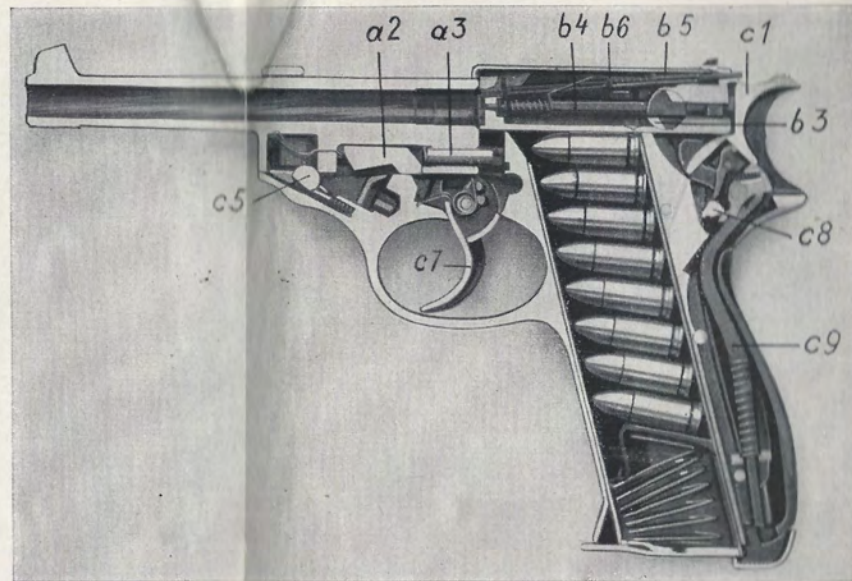
Pistolet 38, aufgeschnitten a 2 Riegel c 1 Hahn a 3 Riegelbolzen c 5 Laufhaltehebel b 3 Sicherung c 7 Abzug b 4 Schlagbolzen c 8 Spannstück b 5 Signallift c 9 Schlagstange mit Feder b 6 Dedel zur Kammer
